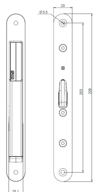
Måttskiss för STEP 535.
